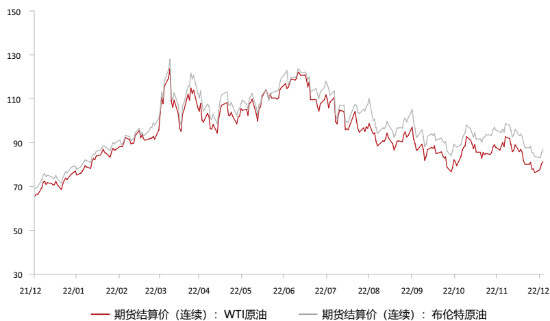
■ 图表 297. 俄乌冲突抬升油价（美元/桶）
